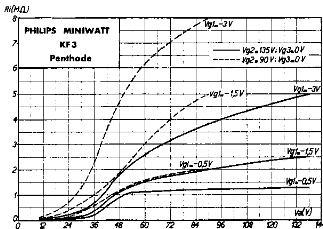
Résistance interne du tube KF 3 en fonction de la tension d'anode pour des tensions négatives de la grille et pour V_{g2} = 135 V et V_{g3} = 90 V.
