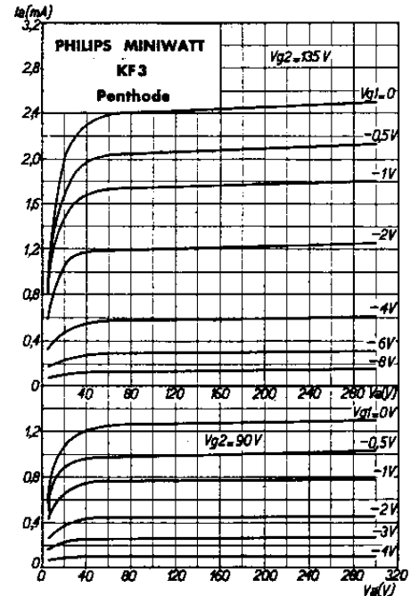
Courant d'anode en fonction de la tension d'anode, pour différentes tensions négatives de la grille et pour V_{g2} = 135 V et V_{g3} = 90 V.
