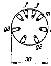
Disposition des électrodes et connexions du culot de la lampe KF 3.
