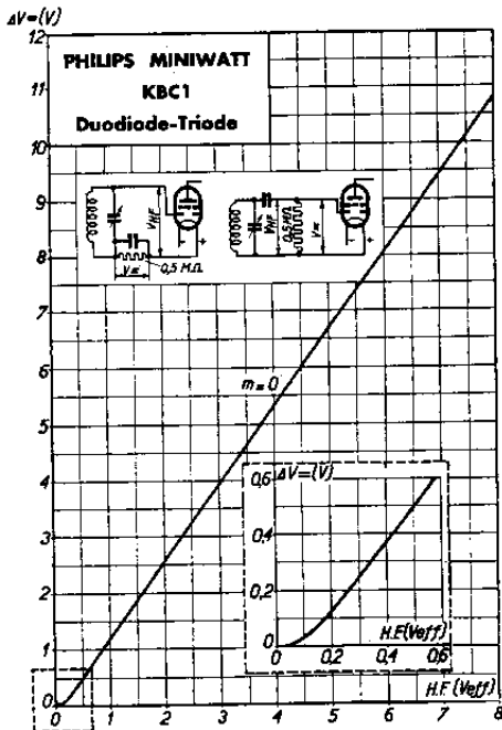
Augmentation de la tension continue ( \Delta V ) aux bornes de la résistance de fuite ( 0,5 M\Omega ) d'une diode de la KBC 1 en fonction de la tension alternative haute fréquence non modulée appliquée à la diode.
