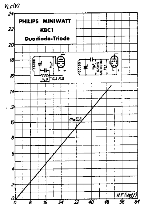
Tension alternative de basse fréquence ( V_{LF} ) aux bornes de la résistance de fuite ( 0,5 M\Omega ) d'une diode du tube KBC 1 en fonction de la tension alternative haute fréquence, modulée à 30%, sur la diode.
