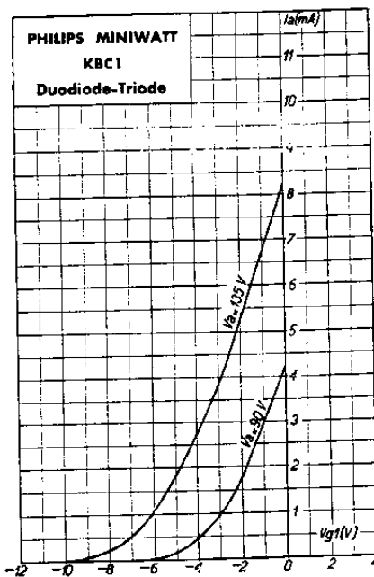
Caractéristiques I_a/V_{g1} de la partie triode du tube KBC 1.
